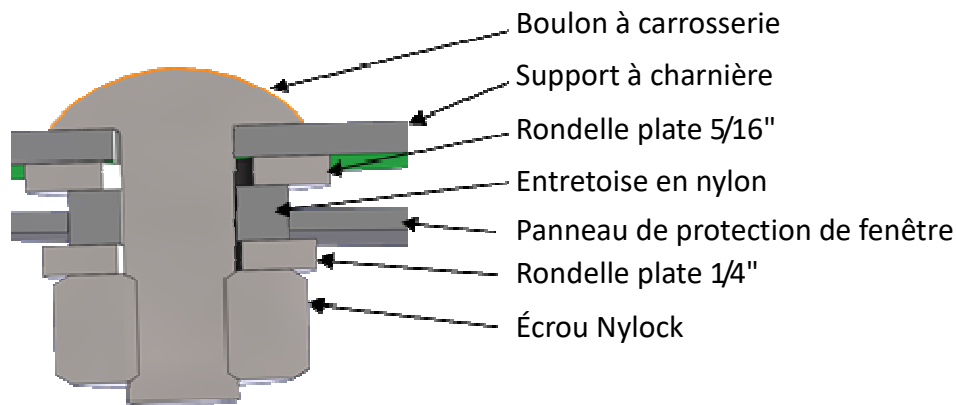
Image 2 - Assemblage de boulon de charnière
